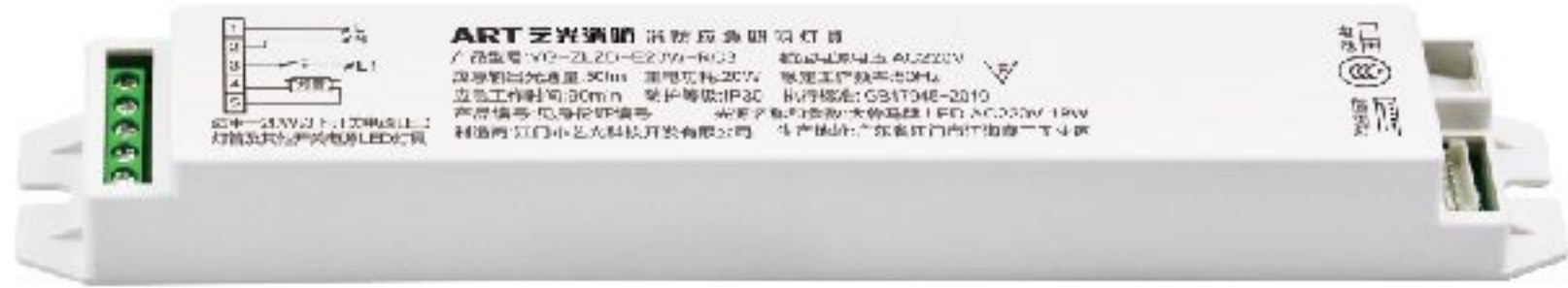
YG-ZLZD-E20W-RC3 订货号：YG-RC3(3000mA/4500mA) 产品尺寸：231x35x25mm 主电功率：20W
